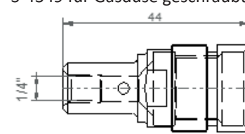
S-4349 für Gasdüse geschraubt
