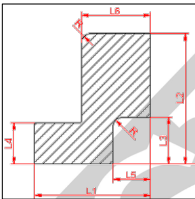
Wirbalit®N Profil 2248
