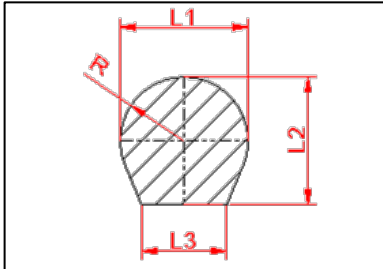
Wirbalit®N Profil 2357
