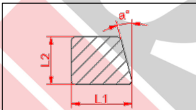
Wirbalit®N Profil 5930
