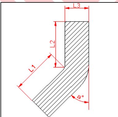
Wirbalit®L Profil 5867
